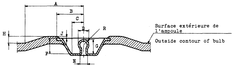
Autre forme du bord du bouton
